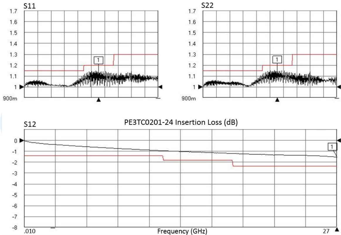
PE3TC0201-24 VSWR
