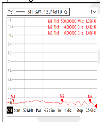
Input VSWR@-40°C
