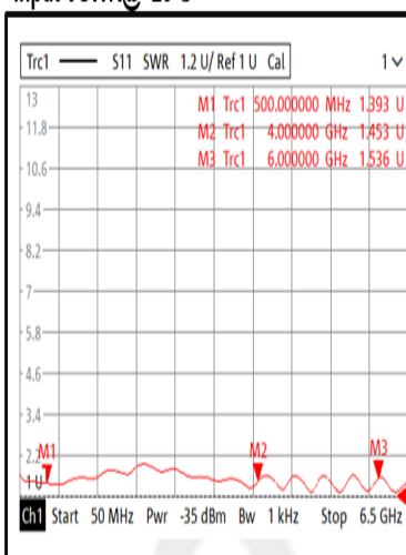
Input VSWR@+25°C
