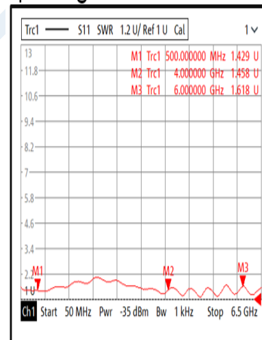
Input VSWR@+85°C
