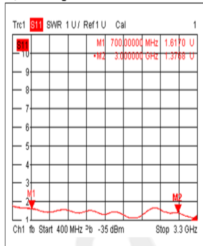
Input VSWR@+25°C
