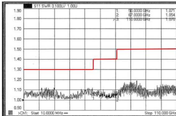
S11 VSWR
