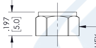
CLAMP NUT
